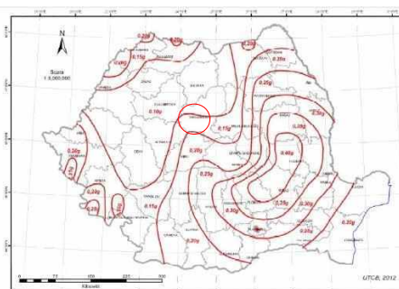
Figura 3.1 România - Zona de valori de vârf ale accelerației terenului pentru proiectare a_g cu T_M=225 ani și 20% probabilitate de depășire în 50 de ani
